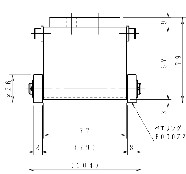
端面図 (S=1/2)
