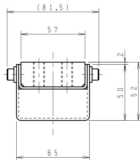
端面図 (S=1/2)
